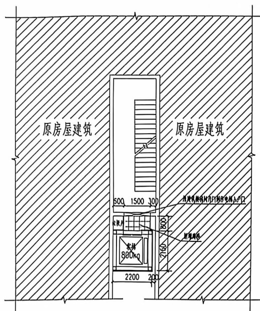
增设电梯标准层平面示意图
