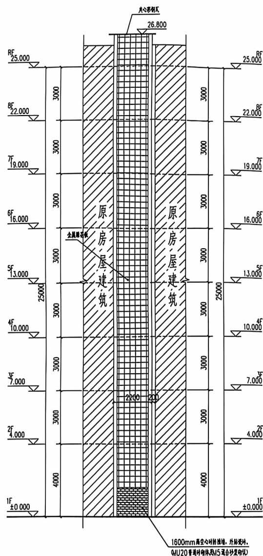
增设电梯立面示意图
