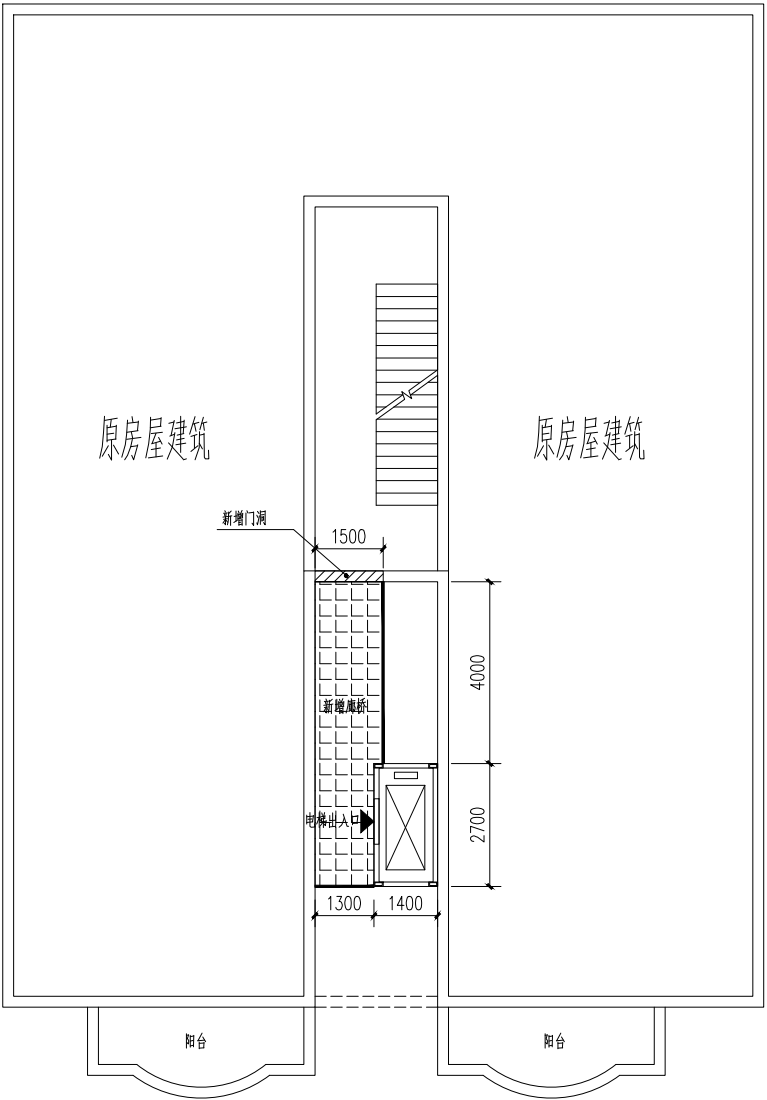
增设电梯标准层示意图 1:100
