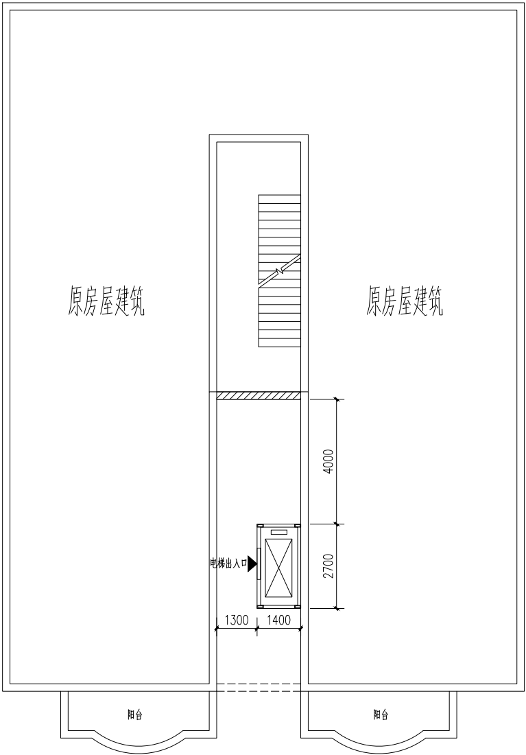
增设电梯一层示意图 1:100
