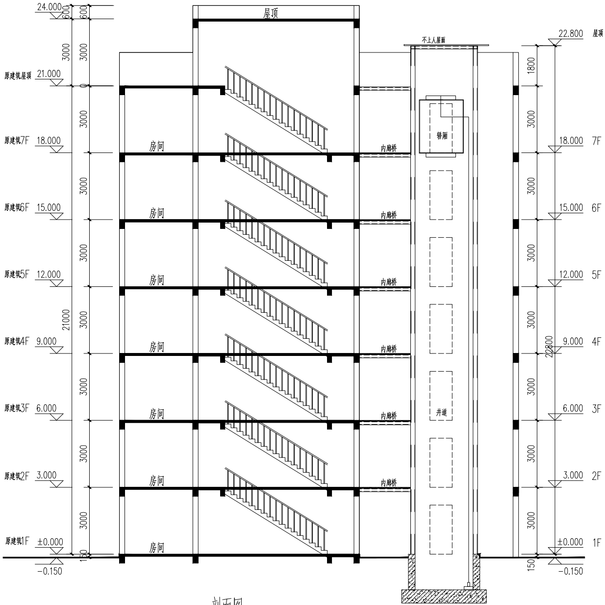
剖面图 1:100
