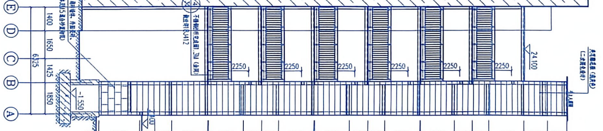
E-A轴立面图 1:100
