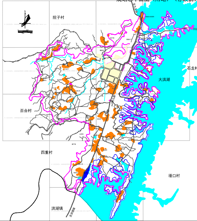
规划总平面图（用地）（修改前）
